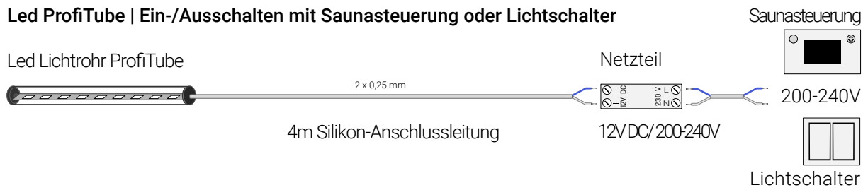
Bild 5 Led ProfiTube | Dimmen mit Saunasteuerung oder Lichtdimmer
