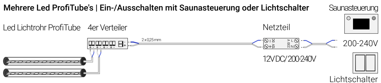
Bild 8 Mehrere Led ProfiTube's | Dimmen mit Saunasteuerung oder Lichtdimmer
