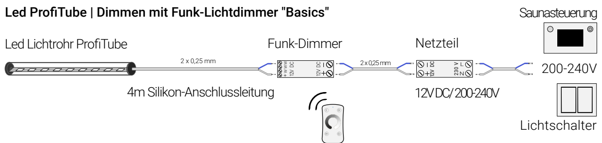
Bild 7 Mehrere Led ProfiTube's | Ein-/Ausschalten mit Saunasteuerung oder Lichtschalter
