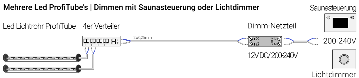
Bild 9 Mehrere Led ProfiTube's | Dimmen mit Funk-Lichtdimmer "Basics"
