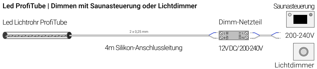
Bild 6 Led ProfiTube | Dimmen mit Funk-Lichtdimmer "Basics"
